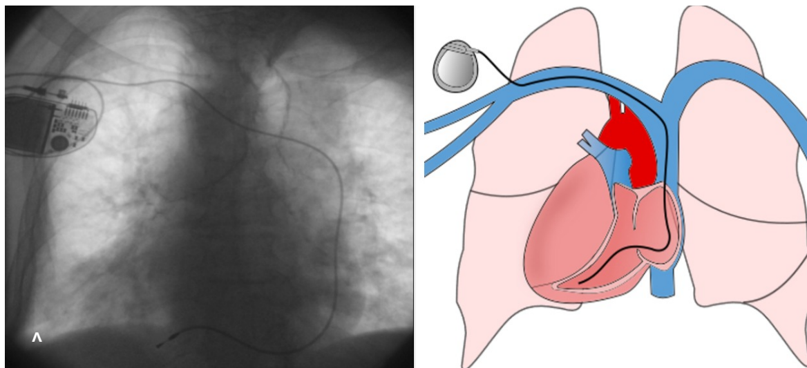
Fig. 1 A) Imagen fluoroscópica con electrodo en ventrículo derecho. Se observa el cable del marcapaso que se introdujo por la vena subclavia derecha, baja por la vena cava superior que está a la izquierda, pasa por la aurícula derecha y termina en el ventrículo derecho. B) Esquema que muestra el trayecto del electrodo bipolar
