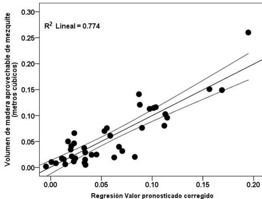
Figura 2. Gráfica de dispersión del volumen cosechable ( m^3 ) de mezquite con ajuste lineal e intervalos de confianza de 95% de la media en Satevó, Chihuahua, México.
