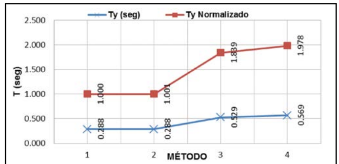
Figura 9. Comparación de periodos en dirección Y y normalización respecto al método estático en edificio sin daños.
